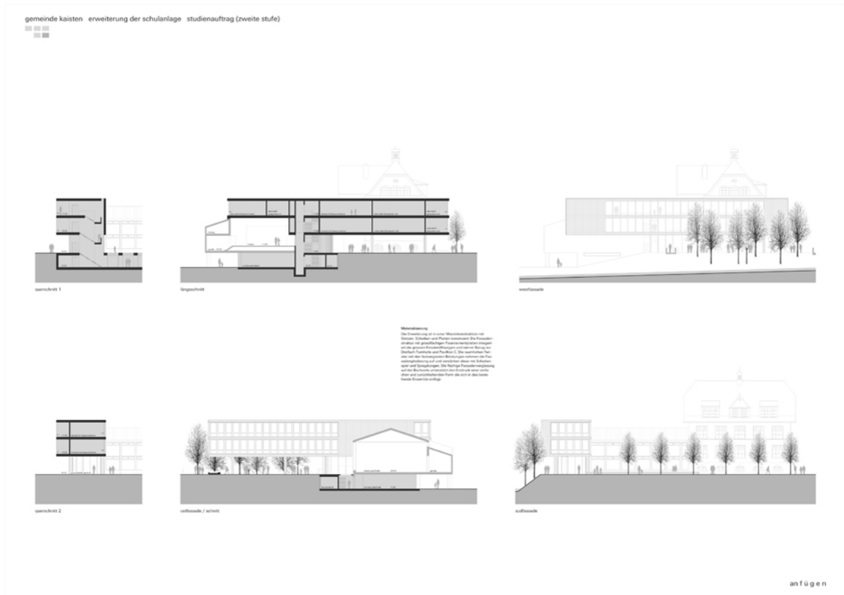
Fassaden / Schnitte
