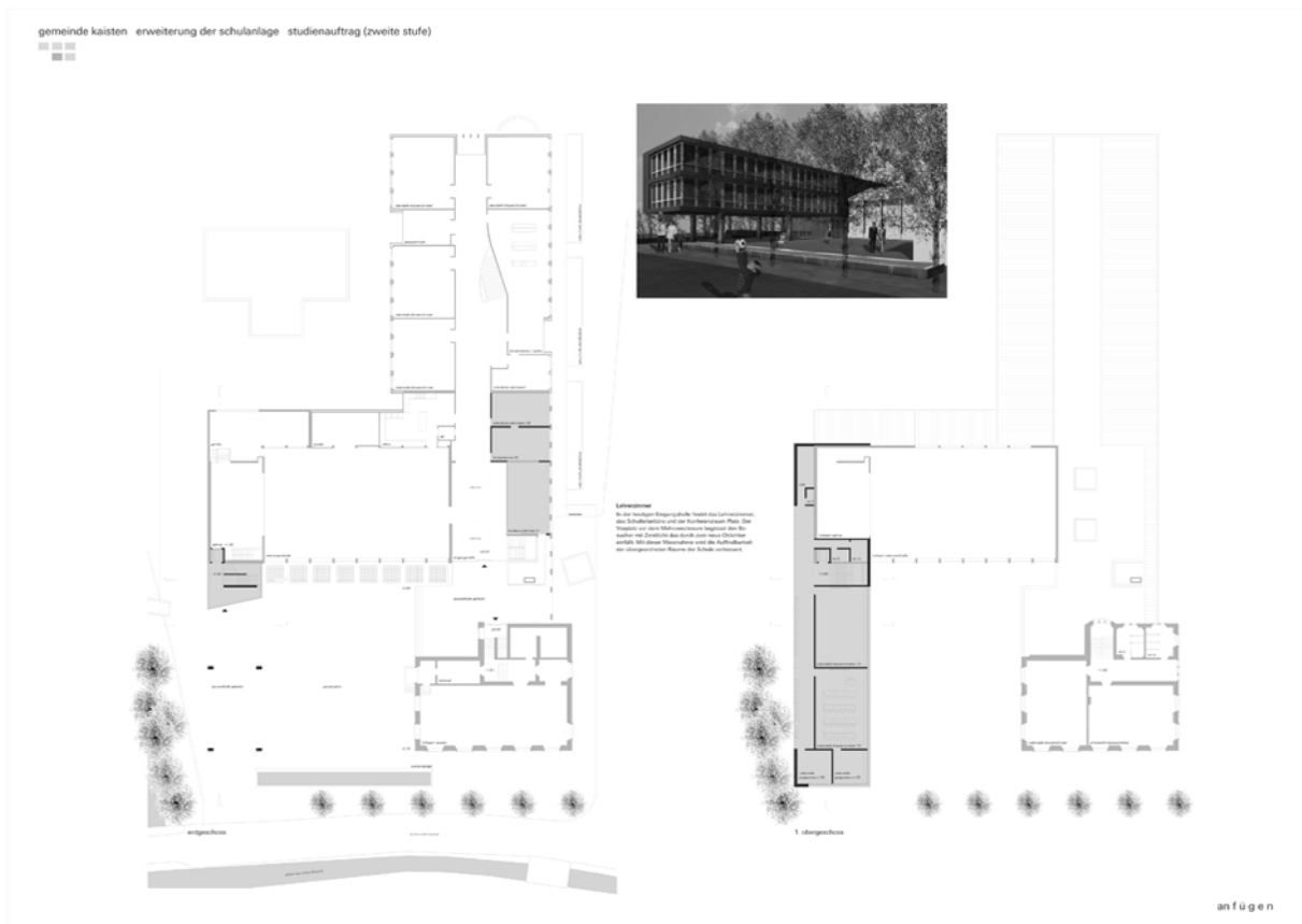
Erdgeschoss / 1. Obergeschoss
