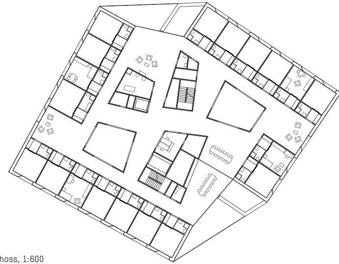
Regelgeschoss, 1:600
